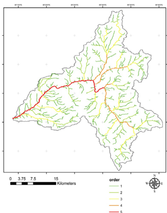
شکل ۷: نقشه هیدروگرافی حوضه رودخانه گیوی چای
