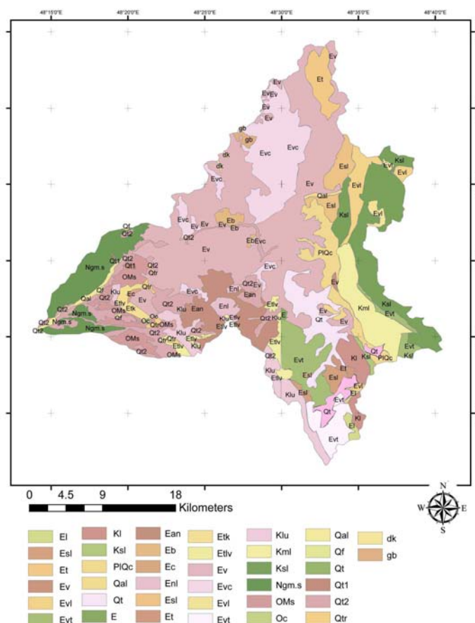
شکل ۵: نقشه لیتولوژی حوضه رودخانه‌ی گیوی چای
