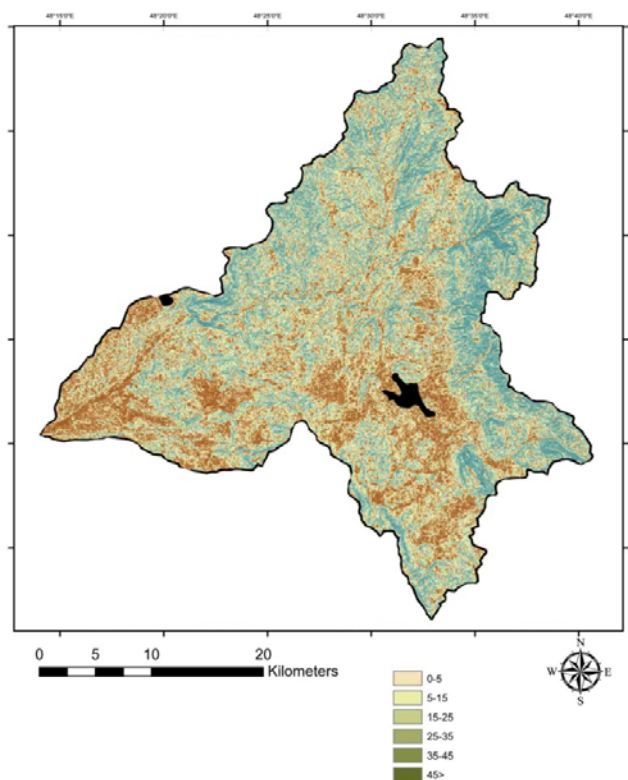
شکل ۲: نقشه شیب در حوضه‌ی رودخانه‌ی گیوی‌چای مأخذ: مطالعات میدانی نگارندگان، ۱۳۹۰
