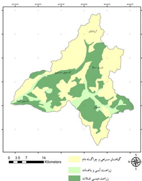
شکل ۸: کاربری اراضی حوضه رودخانه گیوی چای
