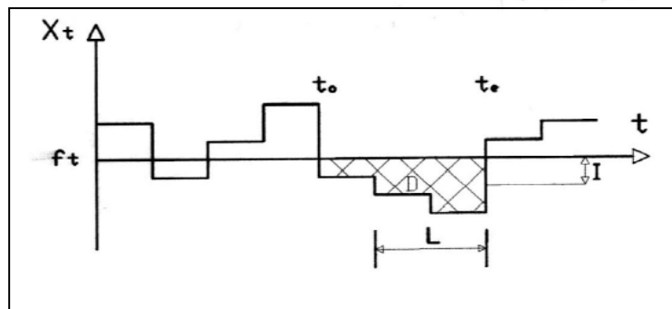
شکل ۱: خصوصیات خشکسالی بر اساس روش ران تست
