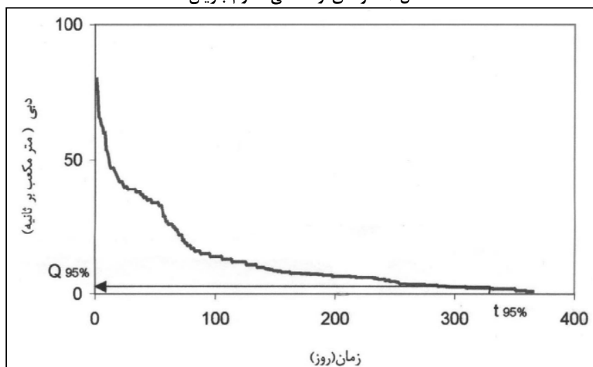
شکل ۲: نمونه‌ای از منحنی تداوم جریان
