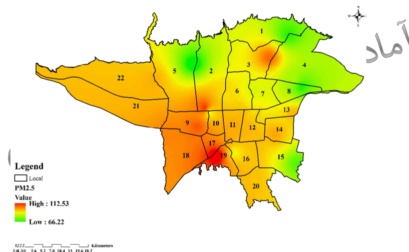
شکل ۵: میزان آلاینده ذرات معلق ( PM_{2.5} ) در کلانشهر تهران در بازه زمانی ۱۳۹۳-۱۴۰۲
