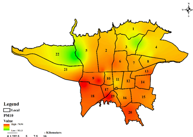
شکل ۶: میزان آلاینده ذرات معلق ( PM_{10} میکرون) در کلانشهر تهران در بازه زمانی ۱۳۹۳-۱۴۰۲
