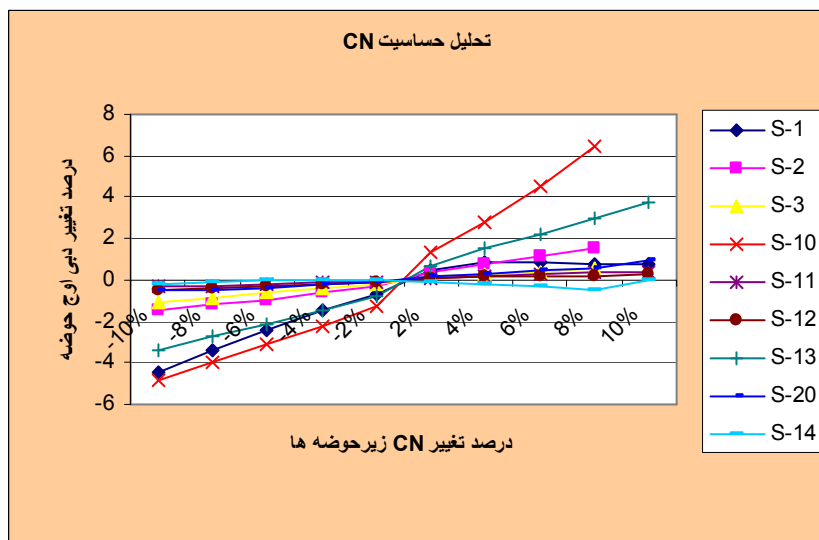
شکل ۷: نمودار آنالیز حساسیت زیرحوضه‌ها به تغییر CN
