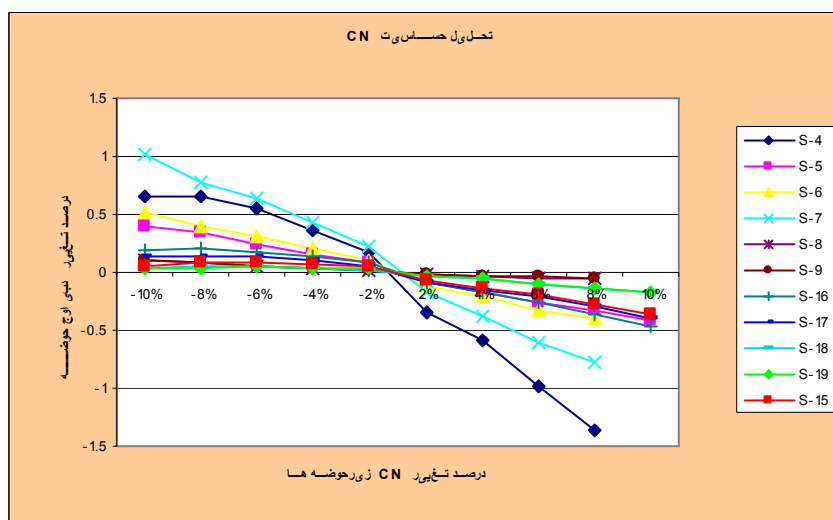
شکل ۸: نمودار آنالیز حساسیت زیرحوضه‌ها به تغییر CN
