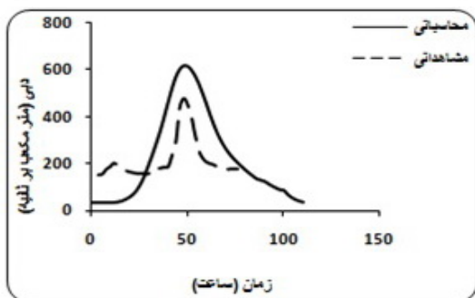
شکل ۳: هیدروگراف مدل قبل و بعد از واسنجی برای سیل ۸۶/۱۱۶ مأخذ: مطالعات میدانی نگارندگان، ۱۳۹۰
