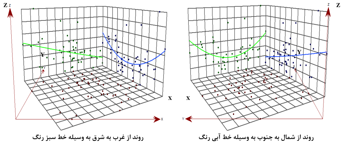
شکل ۳: روند تغییرات شدت خشکسالی استان خراسان رضوی در مرداد ماه ۱۳۷۹ (طول جغرافیایی)
