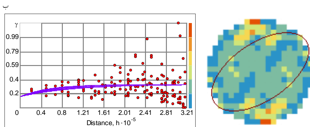
شکل ۴: جهت‌یابی و سمی‌واریوگرام مدل کریجینگ عمومی استان خراسان رضوی (مردادماه ۱۳۷۹) مأخذ: نگارندگان
