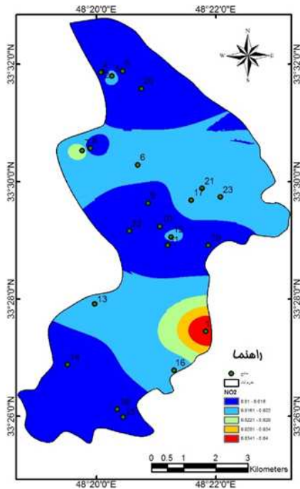
شکل ۳۴: تغییرات NO_2 چاه‌ها و چشمه‌ها در فصل زمستان
