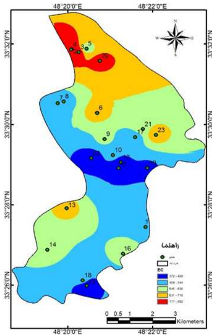
شکل ۱۲: تغییرات EC چاه‌ها و چشمه‌ها در فصل تابستان
