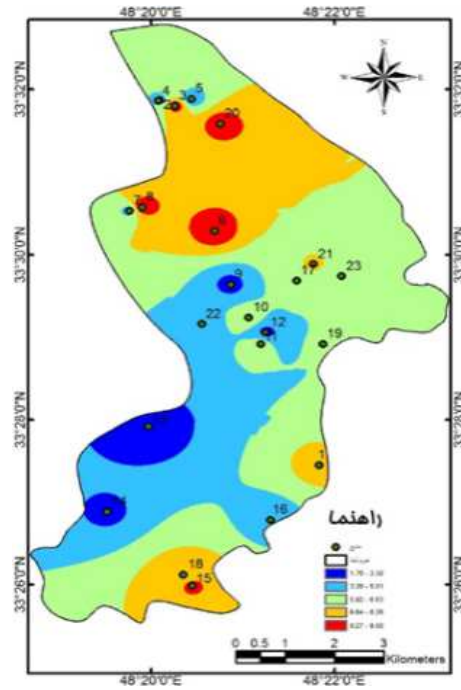
شکل ۲۷: تغییرات NO_3^- چاه‌ها و چشمه‌ها در فصل بهار
