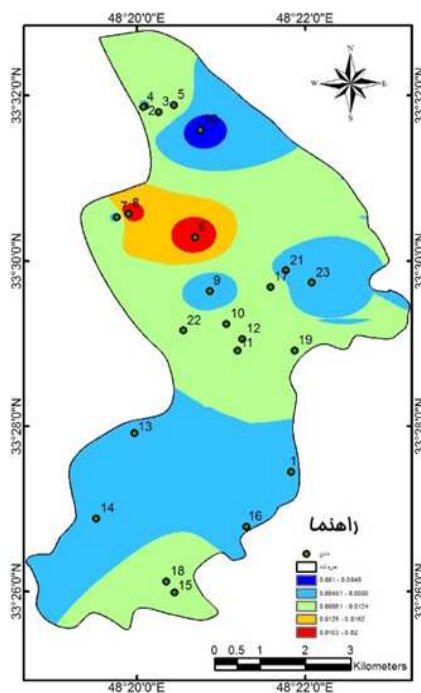
شکل ۳۱: تغییرات NO_2^- چاه‌ها و چشمه‌ها در فصل بهار
