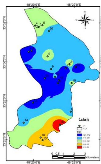
شکل ۲۲: تغییرات SO_4 چاه‌ها و چشمه‌ها در فصل زمستان
