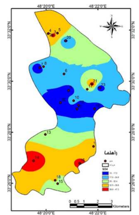
شکل ۲۱: تغییرات SO_4 چاه‌ها و چشمه‌ها در فصل پاییز
