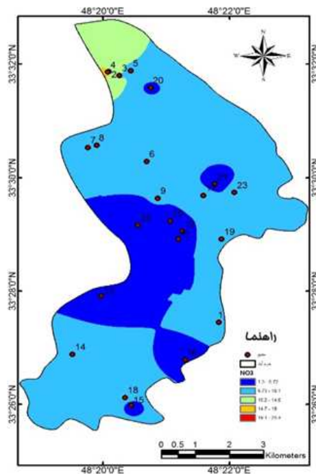
شکل ۲۹: تغییرات NO_3^- چاه‌ها و چشمه‌ها در فصل پاییز
