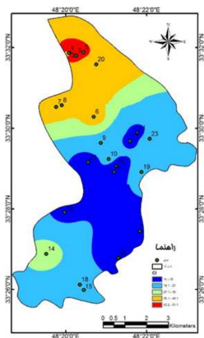
شکل ۲۶: تغییرات NO_3^- چاه‌ها و چشمه‌ها در فصل زمستان
