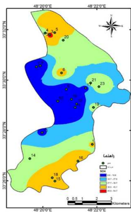
شکل ۲۰: تغییرات SO_4 چاه‌ها و چشمه‌ها در فصل تابستان
