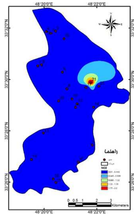
شکل ۳۳: تغییرات NO_2 چاه‌ها و چشمه‌ها در فصل پاییز
