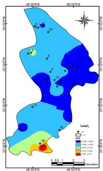
شکل ۳۲: تغییرات NO_2^- چاه‌ها و چشمه‌ها در فصل تابستان
