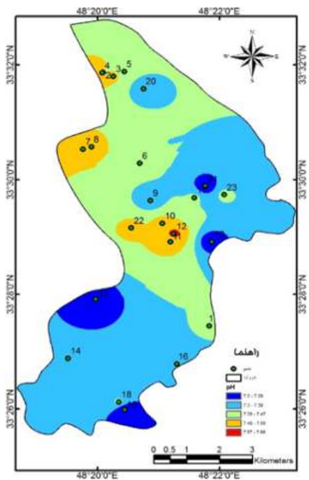
شکل ۴: تغییرات PH چاه‌ها و چشمه‌ها در فصل تابستان
