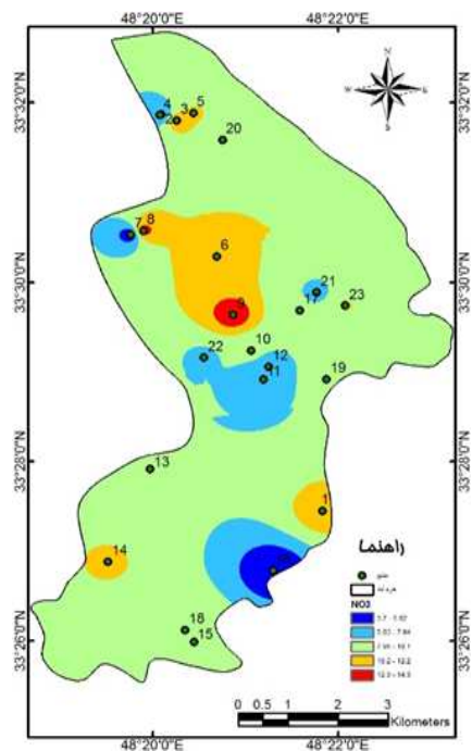
شکل ۳۰: تغییرات NO_3^- چاه‌ها و چشمه‌ها در فصل زمستان
