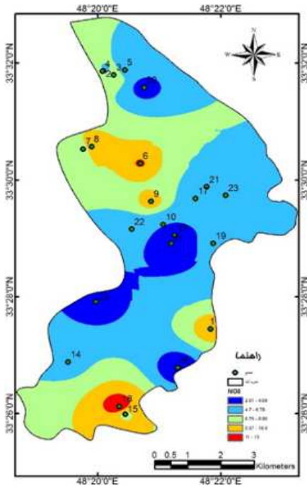
شکل ۲۸: تغییرات NO_3^- چاه‌ها و چشمه‌ها در فصل تابستان
