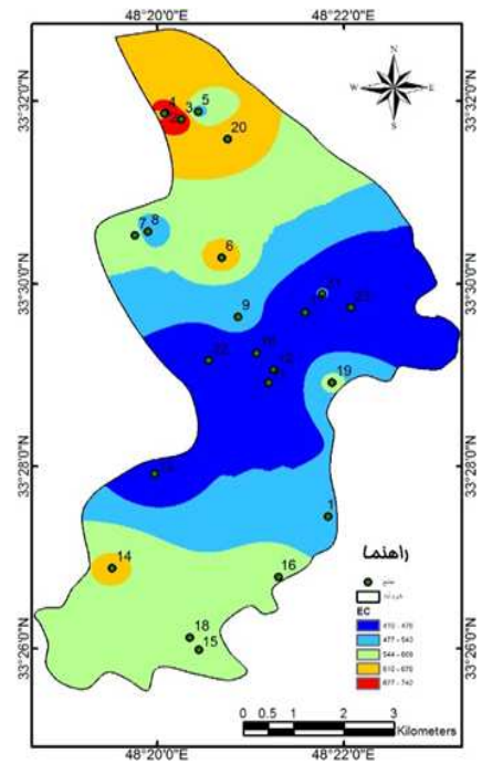
شکل ۱۴: تغییرات EC چاه‌ها و چشمه‌ها در فصل زمستان
