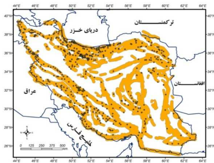
شکل ۱۰: نقشه محدوده بیشینه شتاب لرزه ای g \ 0/4 و بیشتر و موقعیت مراکز جمعیتی مهم قرار گرفته در این پهنه.
