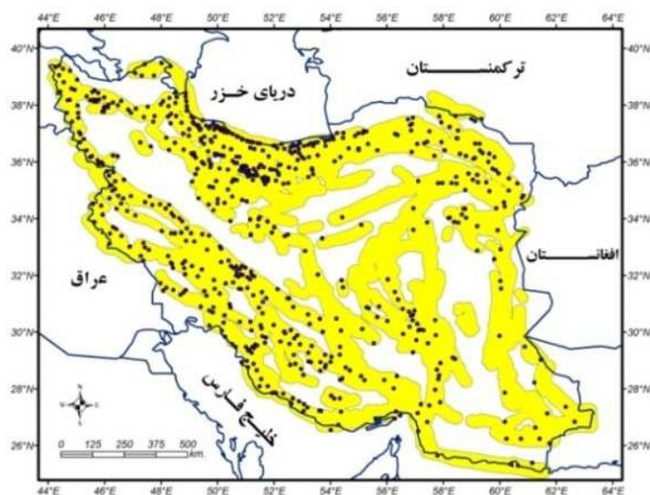
شکل ۹: نقشه محدوده بیشینه شتاب لرزه ای g \ 0/3 و بیشتر و موقعیت مراکز جمعیتی مهم قرار گرفته در این پهنه.
