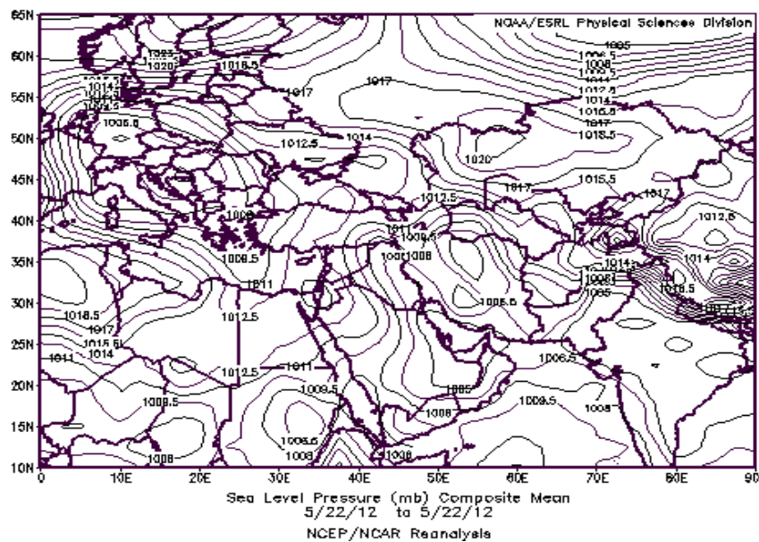
شکل ۳: نقشه فشار سطح دریا
