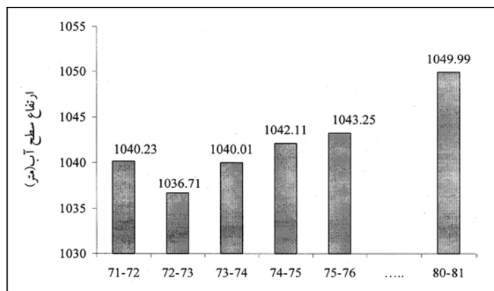
شکل ۱۷: تغییرات ارتفاع آب درچاه پیژومتری نزدیک به حوضچه‌های تغذیه
